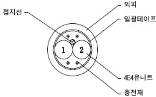
그림1. 구조도
