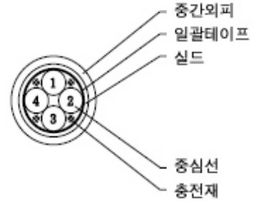
그림2. 4E4유닛 구조도
